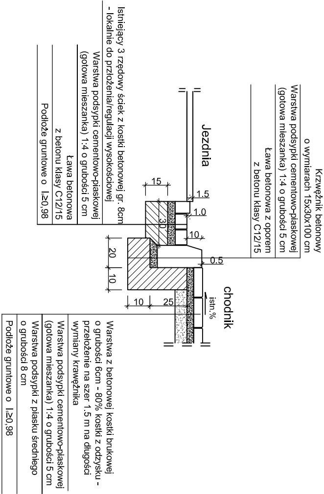
Szczegół A
