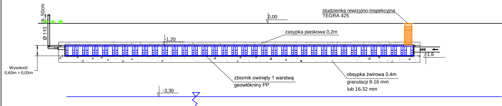
PRZĘKRÓJ A-A
