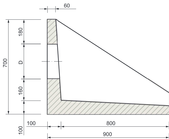
PRZĘKRÓJ 1-1
