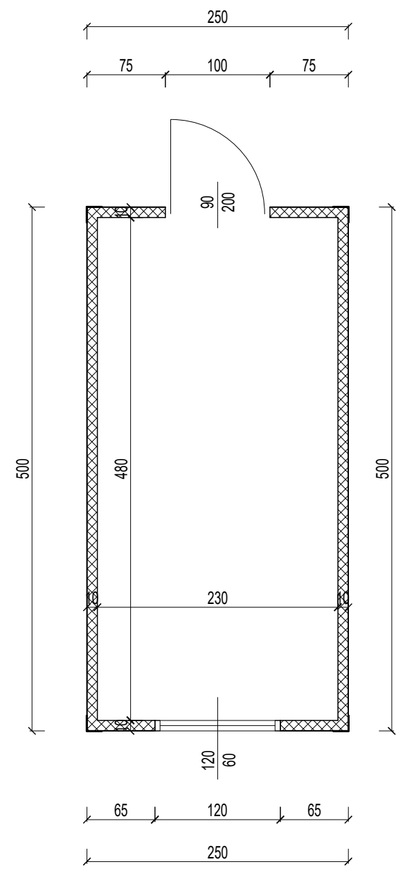
RZUT PRZYZIEMIA 1:50
