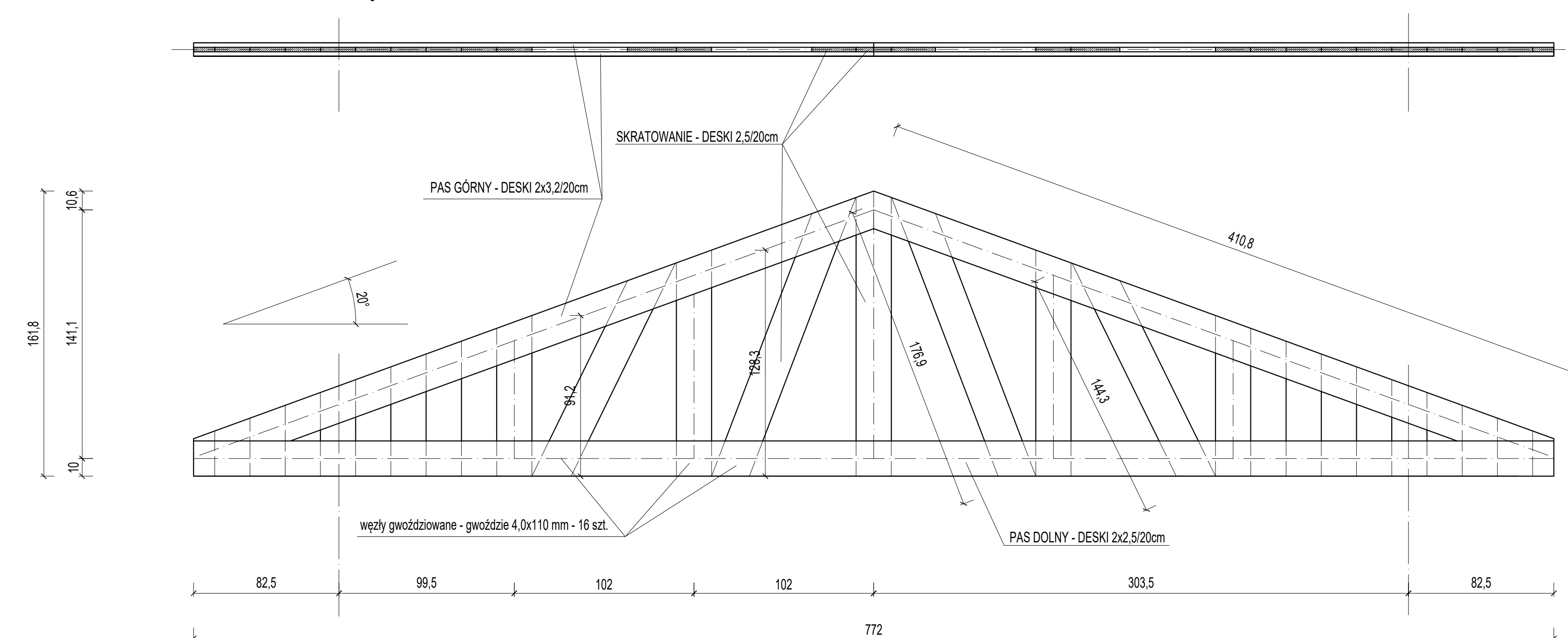
KRATOWY WIĄZAR DESKOWY KWD 2
